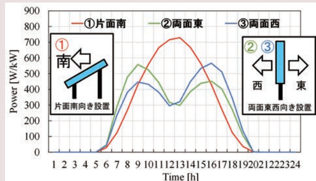
図5 片面受光型と両面受光型太陽電池の出力
