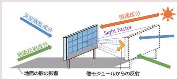
図2 両面受光型太陽電池の発電量推定手法の開発
