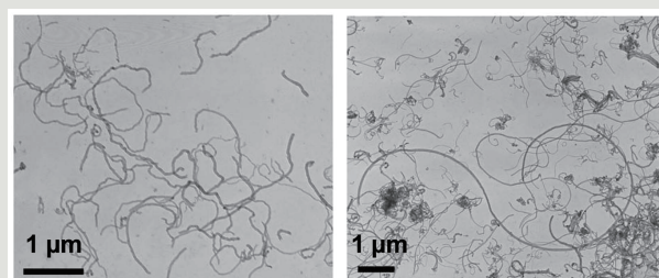
図3 CNTの電子顕微鏡写真
