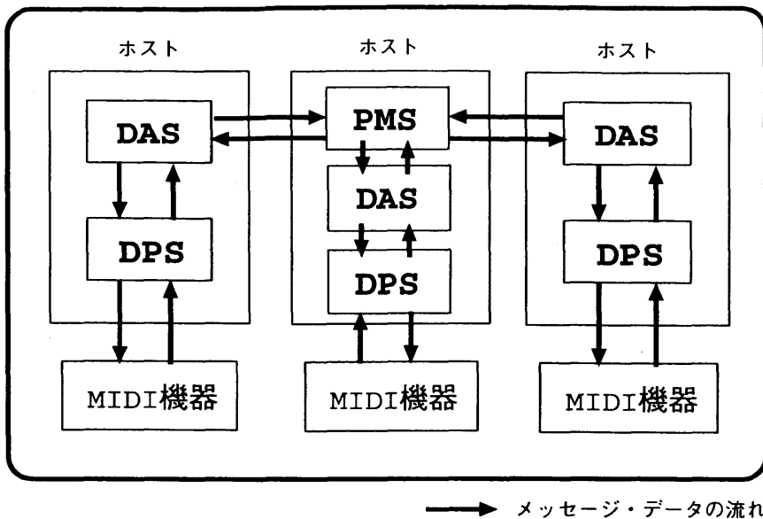
図 3: 実行状態における基本構成図
