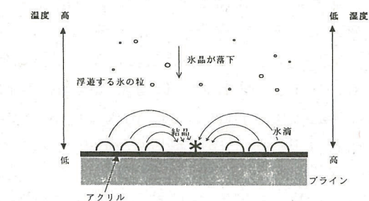
図6： 結晶の成長過程を示す概念図
