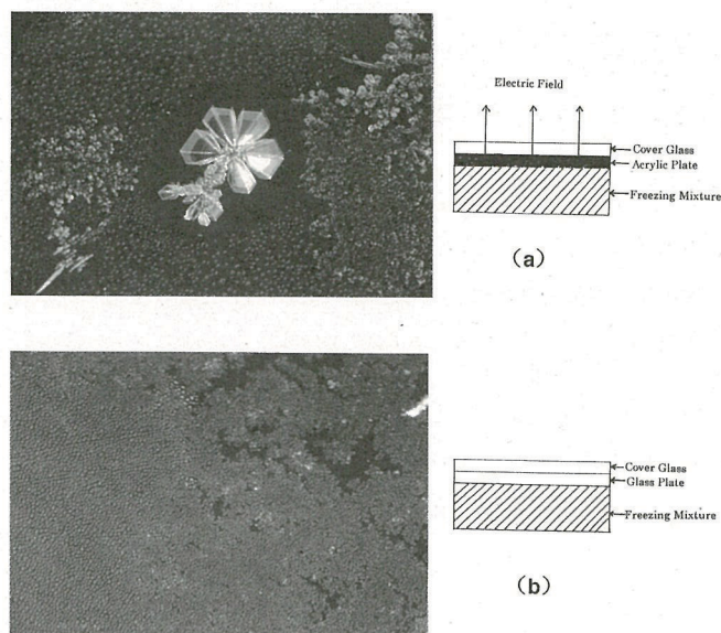
写真11： 結晶成長におよぼす静電気の効果：(a), (b)ともに表面はカバーガラス、(a)はカバーガラスの下に静電気を持つアクリル板が置かれている
