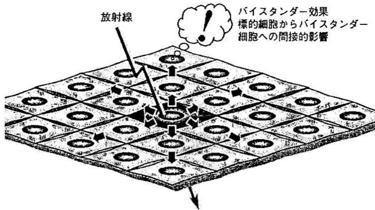
図3 放射線誘発バイスタンダー効果
