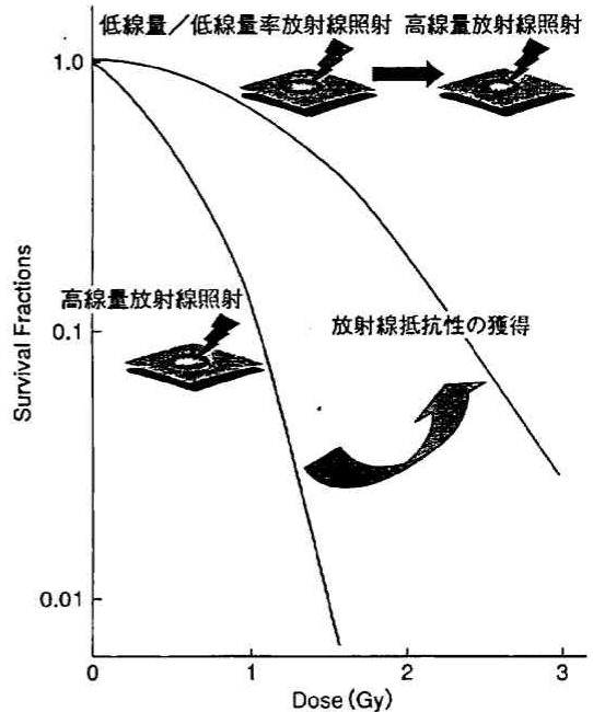
図2 放射線適応応答
