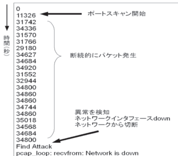
図 11: ポートスキャン時の DTI ハブ動作
