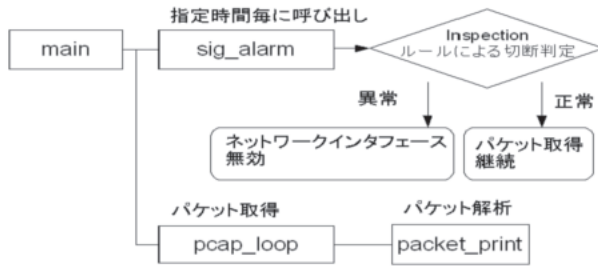
図 6: 関数構造
